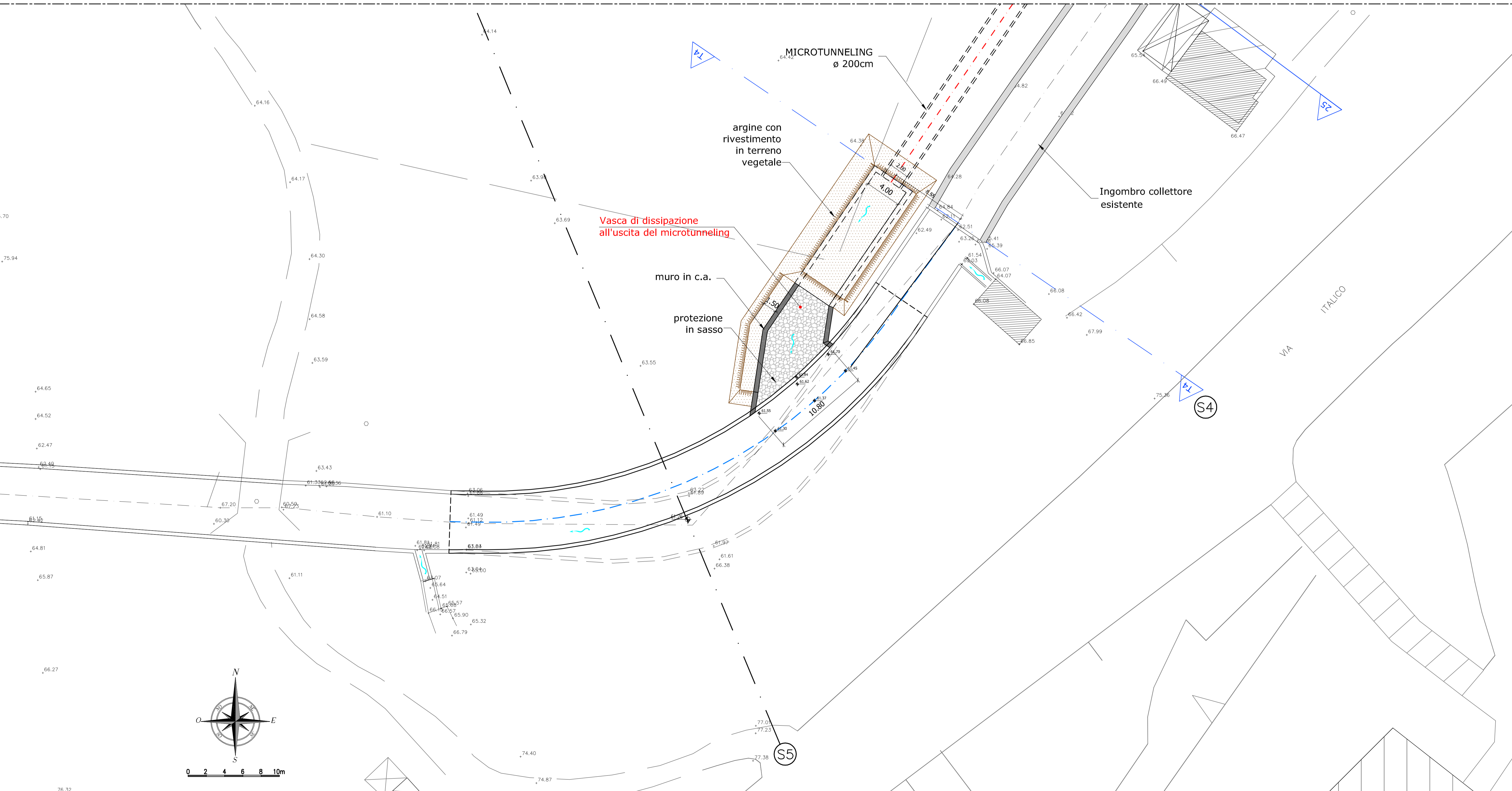
PIANTA SCALA 1:200
